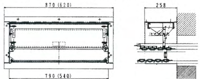
バーコンシャッター ルーピングコンベア用 T750 (T500)
